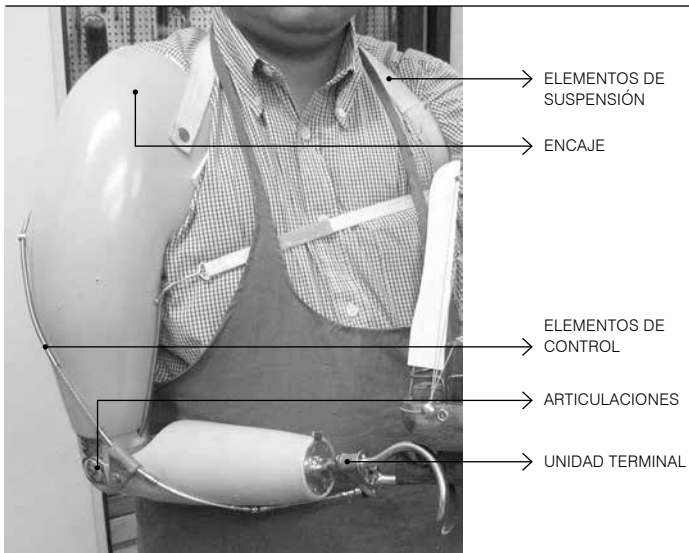
Fig. 12–7. Elementos de una prótesis de miembro superior.
